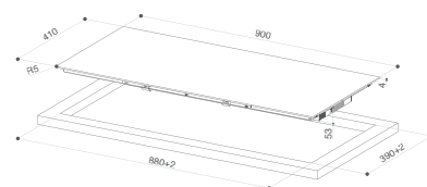
STANDARDNA UGRADNJA
