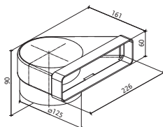
KOLJENO CRCV 90 REVERZIBILNO FUN 112.0157.298
