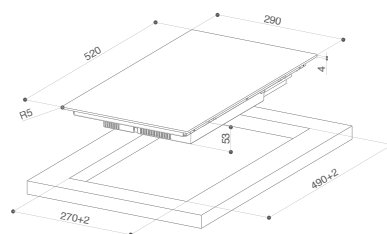
STANDARDNA UGRADNJA
