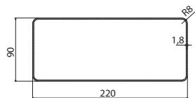
PRAVOKUTNA CIJEV TR 1200 220X90 MM FUN 112.0459.427
