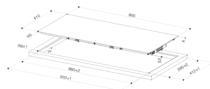
PORAVNANA UGRADNJA
