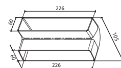
PRAVOKUTNA REDUKCIJA 60H FUN 112.0557.017
