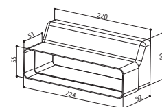
PRAVOKUTNA REDUKCIJA 60H FUN 112.0557.017
