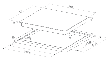
PORAVNANA UGRADNJA
