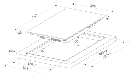
PORAVNANA UGRADNJA
