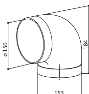
KOLJENO TONDA 90° D150 FUN 112.0253.688
