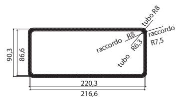
PRAVOKUTNA SPOJNICA 220X90 MM FUN 112.0459.428
