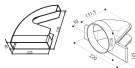
KOLJENO CRCO 90 REVERZIBILNO FUN 112.0157.306
