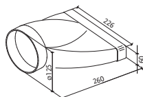
KOLJENO CRCV 90 REVERZIBILNO FUN 112.0157.298
