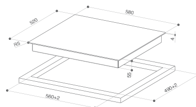
STANDARDNA UGRADNJA
