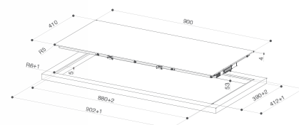
PORAVNANA UGRADNJA
