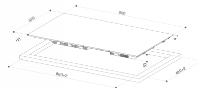
STANDARDNA UGRADNJA
