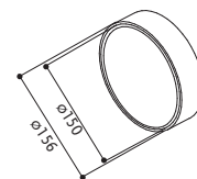
CIJEV TCF 150 L=1,5 M. FUN 112.0280.687
