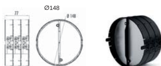
NEPOVRATNI VENTIL 3D D150 FUN 112.0569.781
