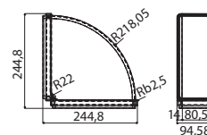
CIJEV TC 1000 Ø 150 MM FUN 112.0253.681
