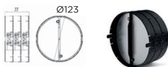
NEPOVRATNI VENTIL 3D D125 FUN 112.0569.782
