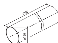
CIJEV TC 1000 Ø 150 MM FUN 112.0253.681
