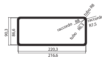
PRAVOKUTNA SPOJNICA 220X90 MM FUN 112.0459.428
