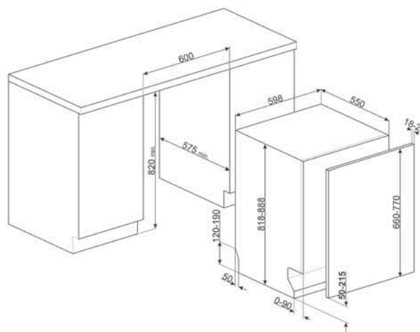
PERILICE POSUĐA ŠIRINE 60 CM, VISINE 82 CM: STL7324AQL, STL7322BQL, STL7322BL, STL7332CL, STL5322BQL, STL7332C, STL5352C, STL273C, STL362DQ
