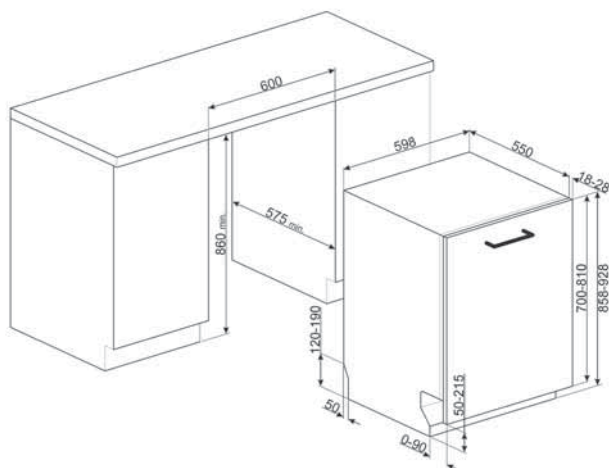
PERILICA POSUĐA ŠIRINE 60 CM, VISINE 86 CM: STL323BQLH
