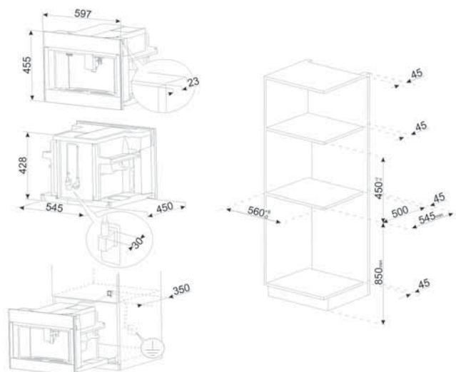
APARATI ZA KAVU: CMS4604NR, CMS4104G
