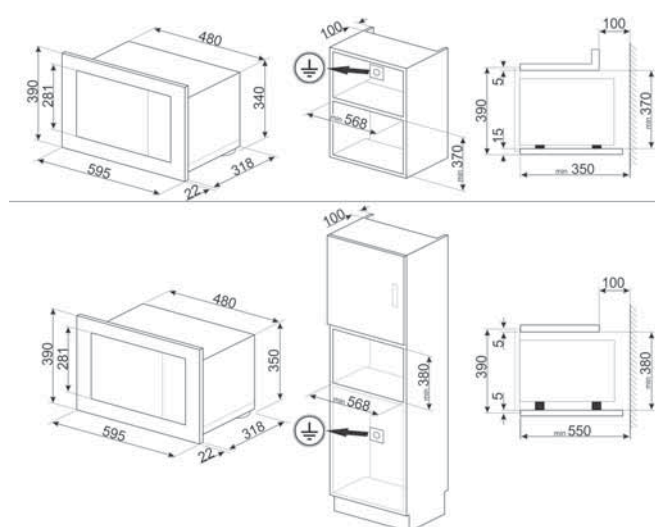
MIKROVALNA PEČNICA: FMI320X2
