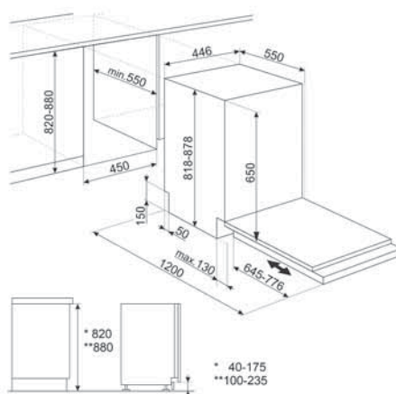
PERILICE POSUĐA ŠIRINE 45 CM, VISINE 82 CM: ST4533IN, ST4523IN, ST4522IN
